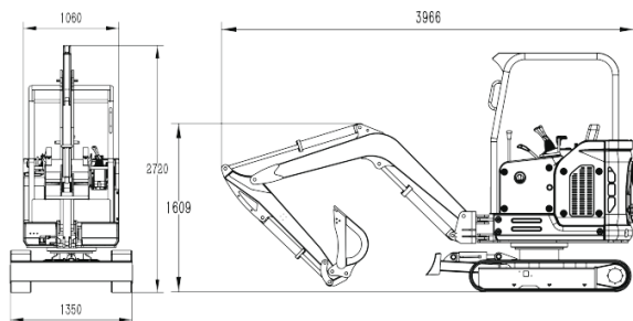
VISTA FRONTAL Y LATERAL · COTAS EN MM
